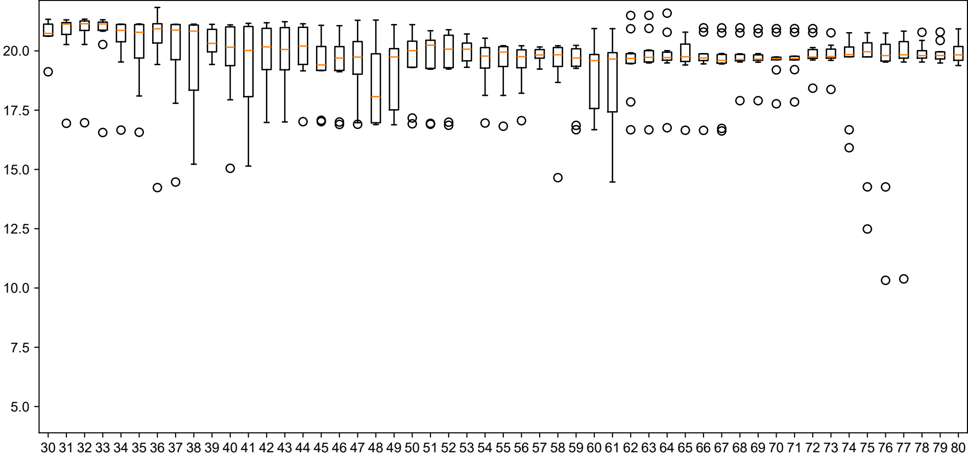
nn
