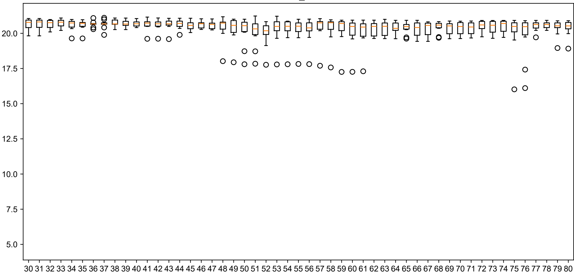
lasso
