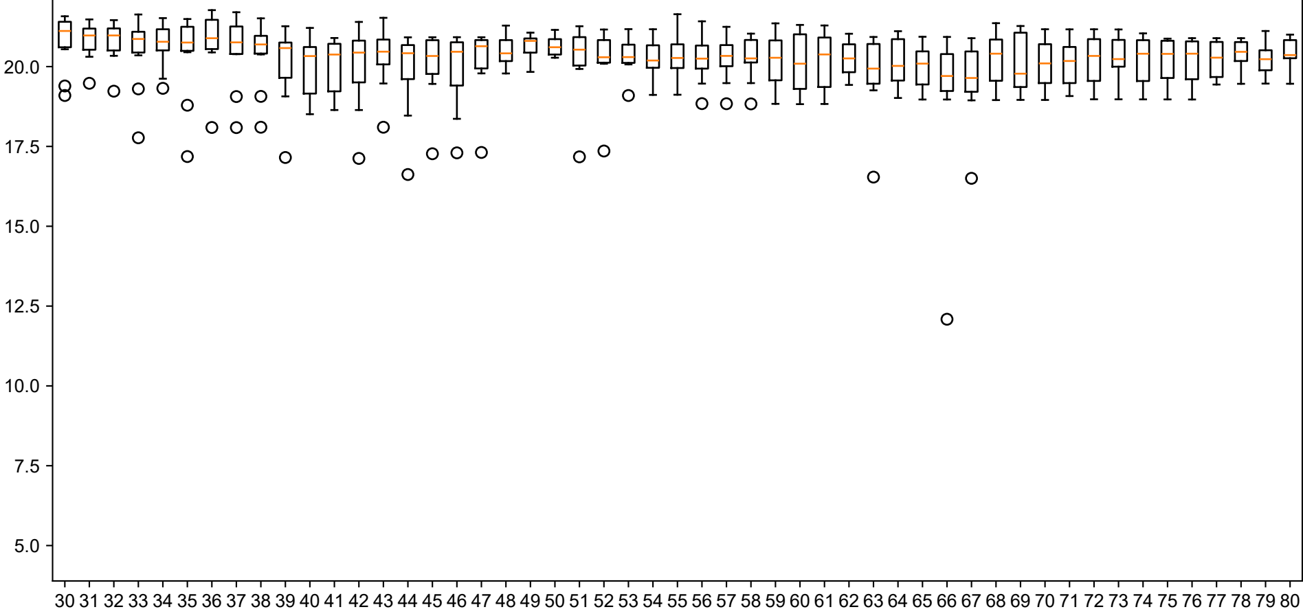
nn
