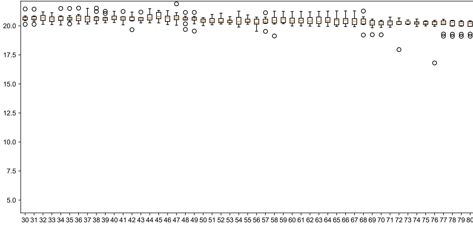
elastic_net
